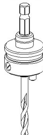
Arbre Starrett A10 avec foret (pour 1 1/2" à 4")
