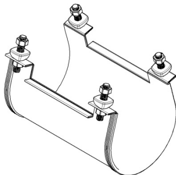
Sangle large avec ses rotules, écrous et goujons.
