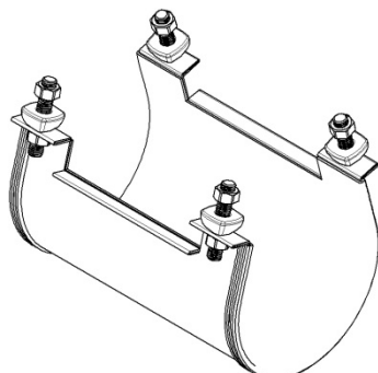
Banda ancha con sus rótulas, tuercas y espárragos.
